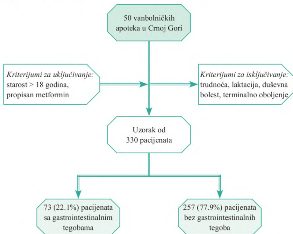
Slika 4. Dijagram toka studije preseka.
