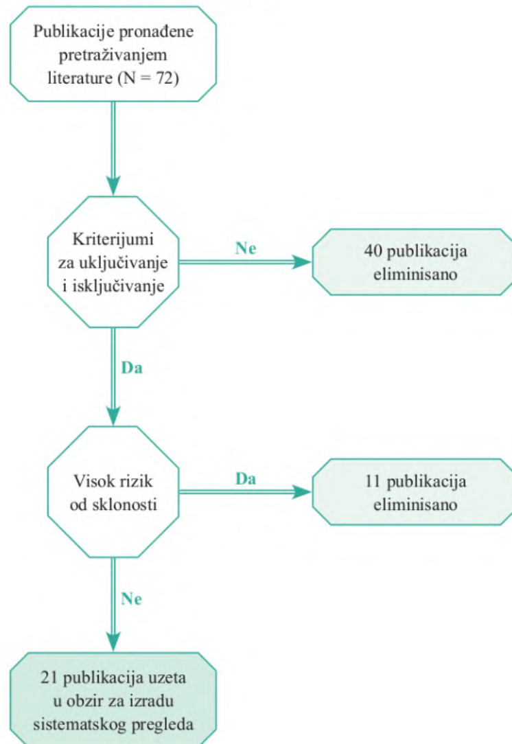
Slika 1. Dijagram toka pronalaženja i selekcije publikacija.
